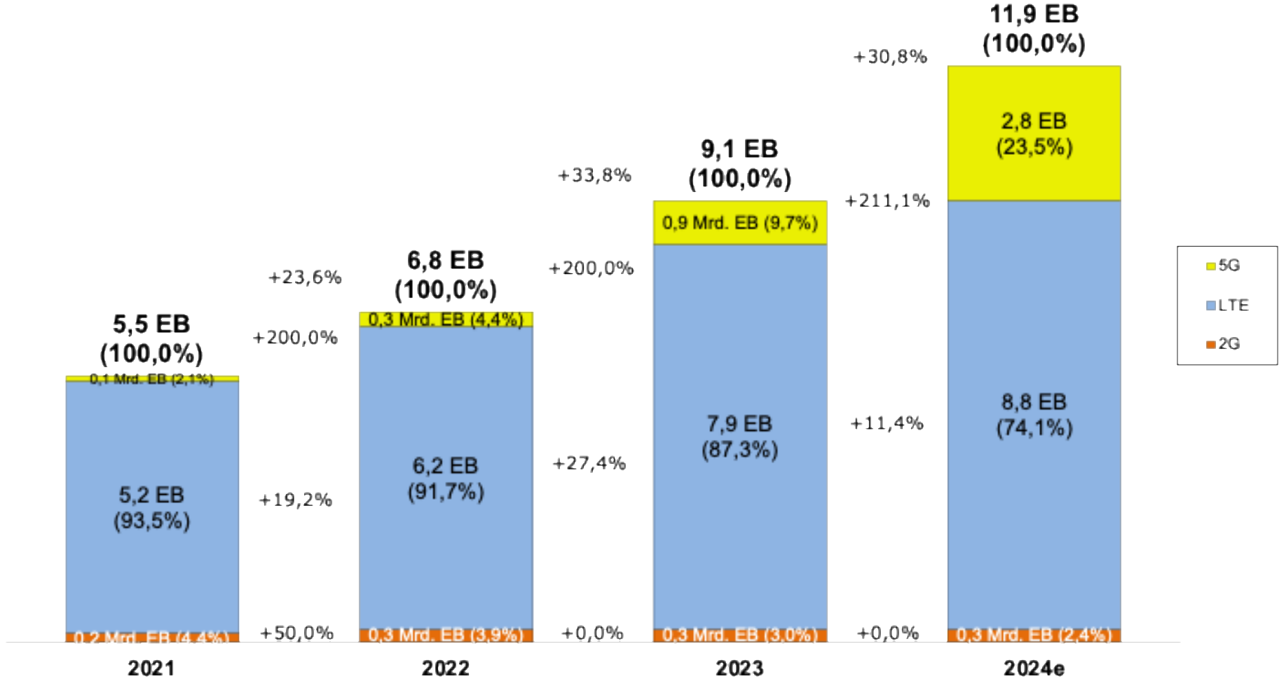
Volumenentwicklung a Datenverkehr aus Mobilfunknetzen nach Technologie
